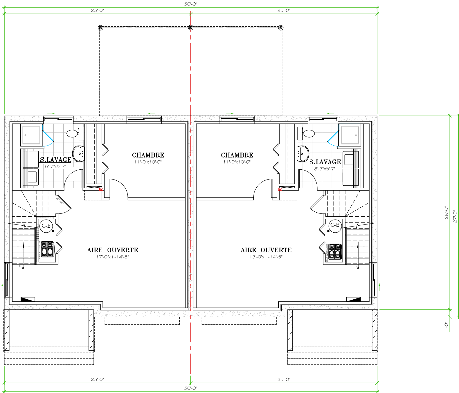
VUE EN PLAN DES FONDATIONS
