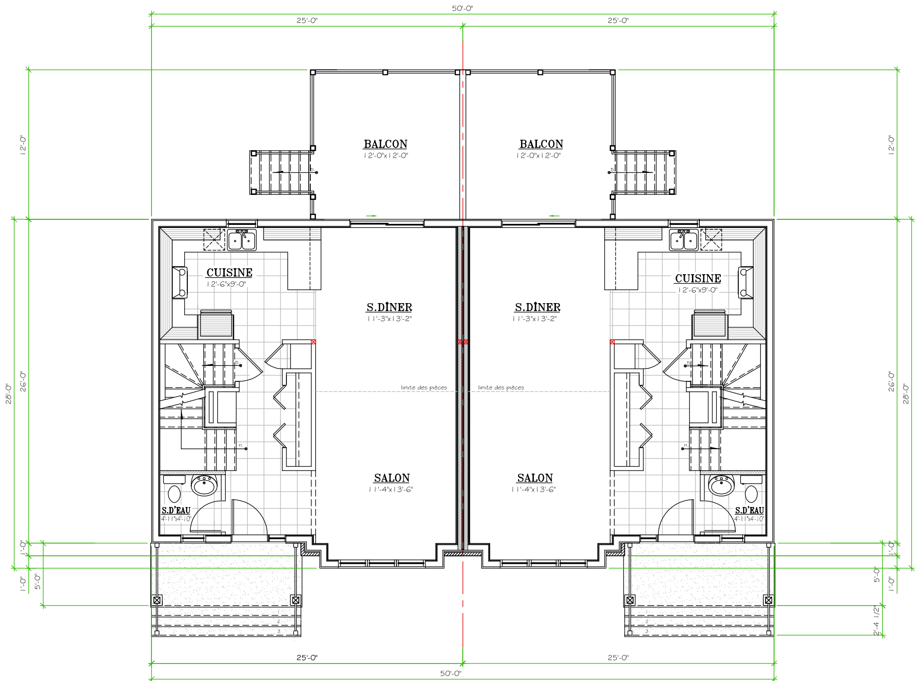
VUE EN PLAN DU REZ-DE-CHAUSSÉE
