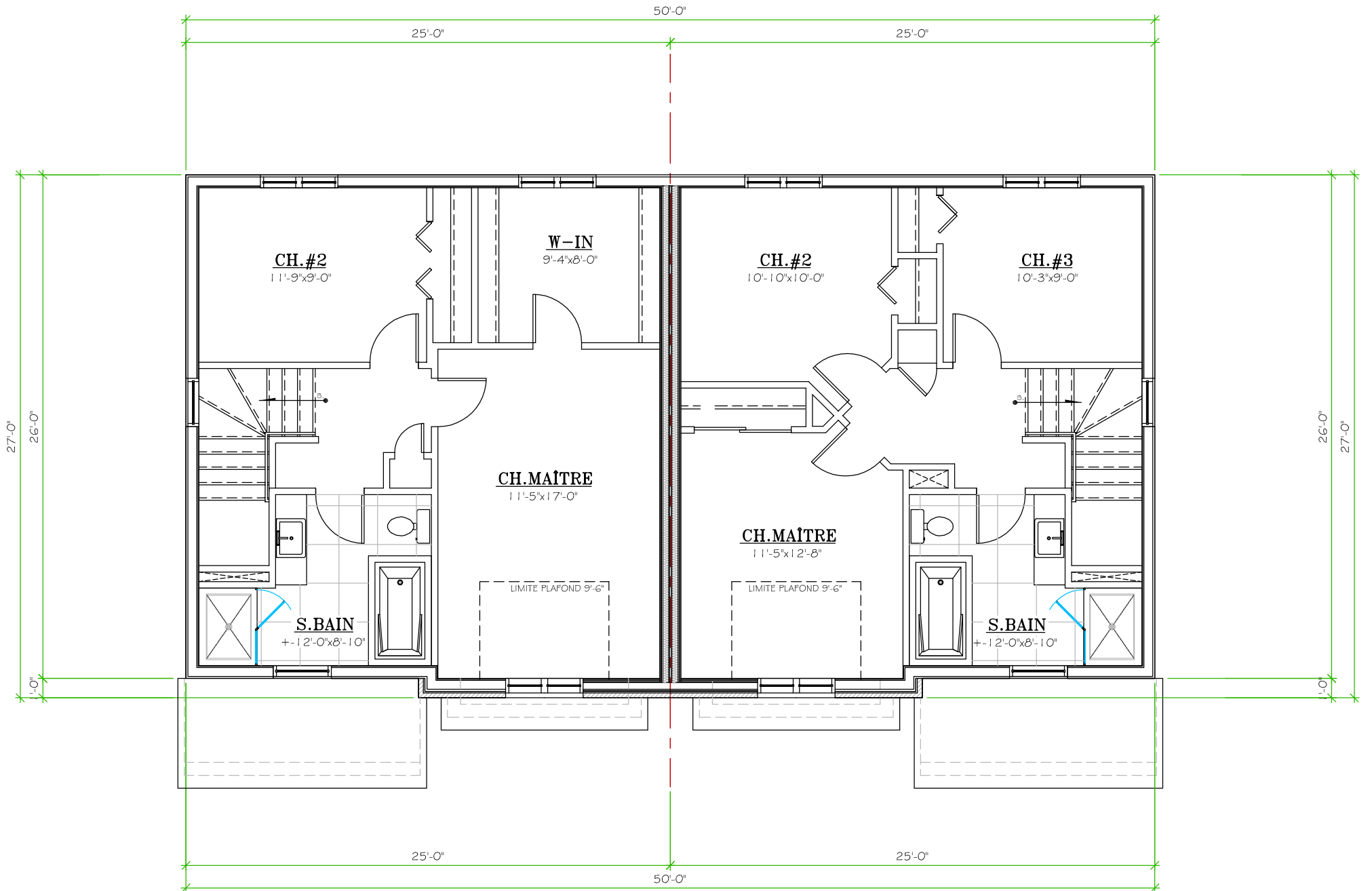
VUE EN PLAN DE L'ÉTAGE
